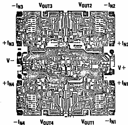
DIE SIZE: 101 x 95 MILS
