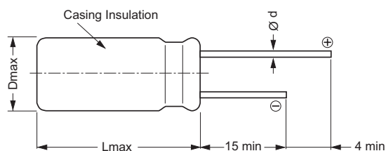
5 ≤ ØD ≤ 18 Long leads EKS 00...
