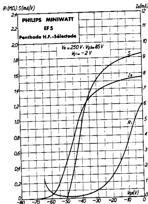
Résistance interne R_i , pente S et courant d'anode I_a en fonction de la tension négative sur la grille 3 pour V_a = 250 \text{ V} , V_{g2} = 85 \text{ V} et V_{g1} = -2 \text{ V} . Fig. 10
