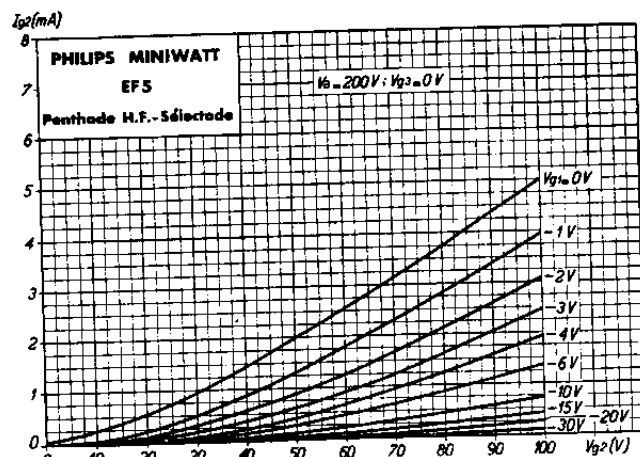
Courant de grille-écran en fonction de la tension sur la grille-écran pour différentes tensions sur la grille de commande. Ces courbes sont approximativement valables pour toutes les tensions d'anode entre 100 et 250 volts.
