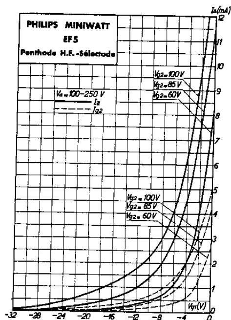
Courant plaque et courant de grille-écran en fonction de la tension de la grille de commande pour 3 tensions différentes de grille-écran et pour une tension d'anode de 250 volts. Les courbes sont approximativement valables pour toutes les tensions d'anode entre 100 et 250 volts.
