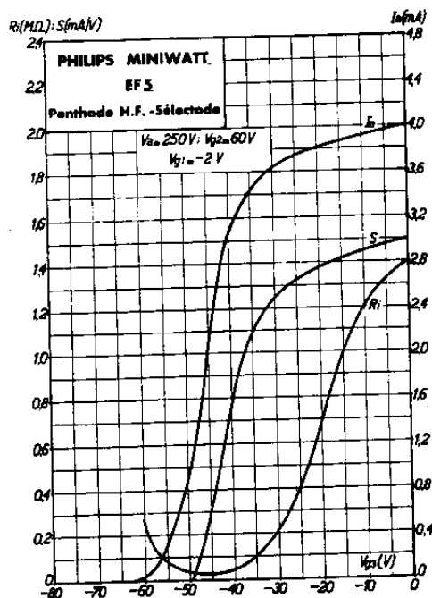
Résistance interne R_i , pente S et courant d'anode I_a en fonction de la tension négative sur la grille 3 pour V_a = 250 \text{ V} , V_{g2} = 60 \text{ V} et V_{g1} = -2 \text{ V} . Fig. 11
