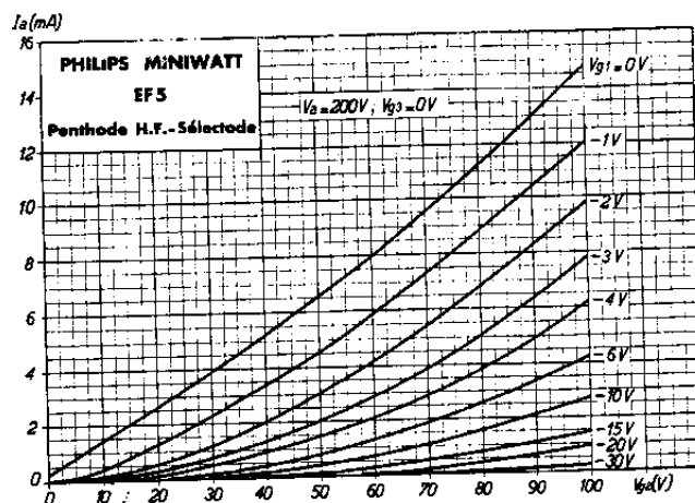
Courant d'anode en fonction de la tension sur la grille-écran pour différentes tensions sur la grille de commande. Ces courbes sont approximativement valables pour toutes les tensions d'anode comprises entre 100 et 250 volts.
