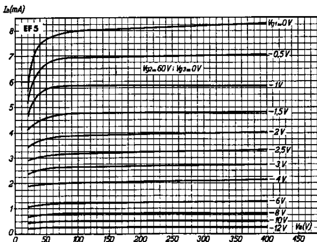
Courant plaque en fonction de la tension plaque pour différentes polarisations négatives de la grille de commande et pour 3 tensions différentes de grille-écran.
