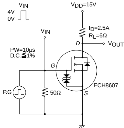
スイッチングタイム測定回路図
