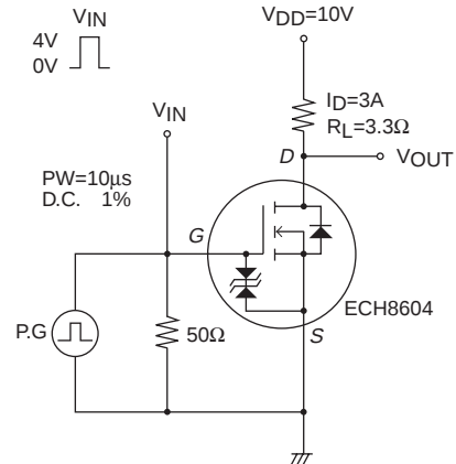
スイッチングタイム測定回路図
