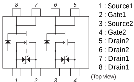
電氣的接続図
