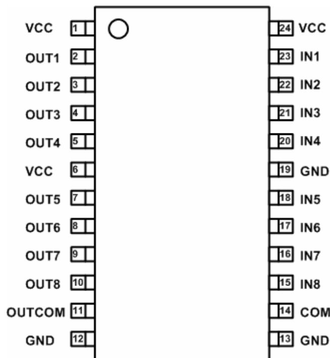
SSOP – 24
