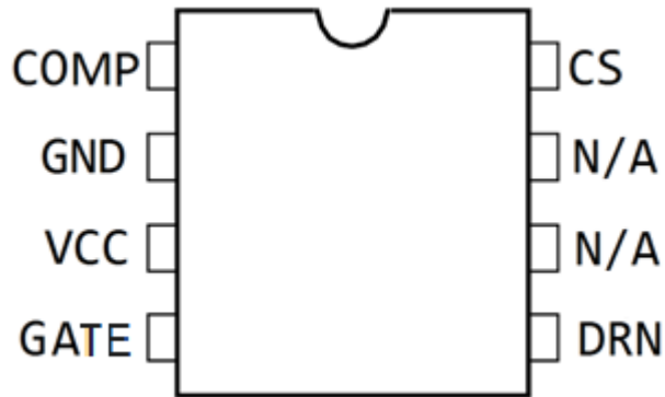
SOP8 封装
