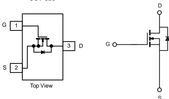
SOT-323
