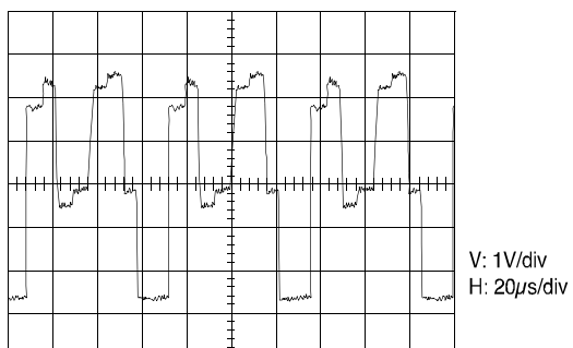
(1) I101 PIN 19
