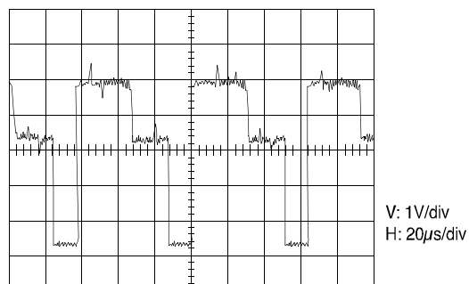
(2) I101 PIN 20
