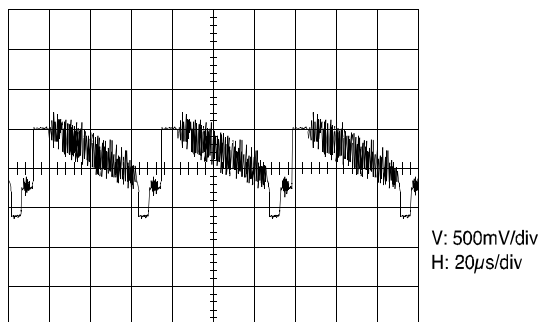
(5) I101 PIN 44
