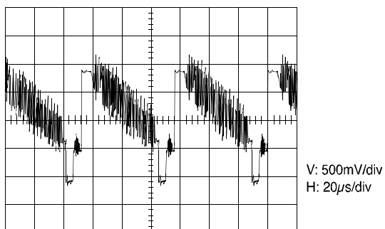
(5) I101 PIN 40
