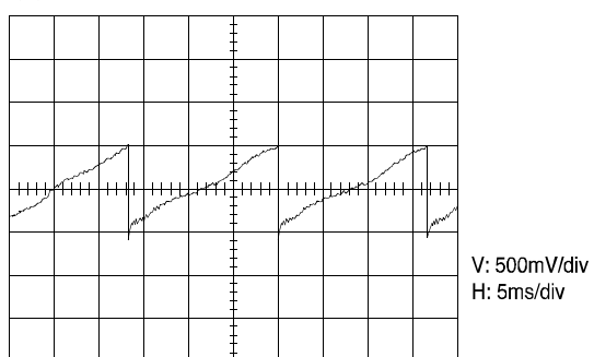
(4) I101 PIN 23
