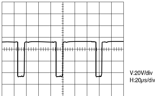
1) I701 PIN 18
