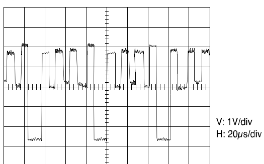
(3) I101 PIN 21
