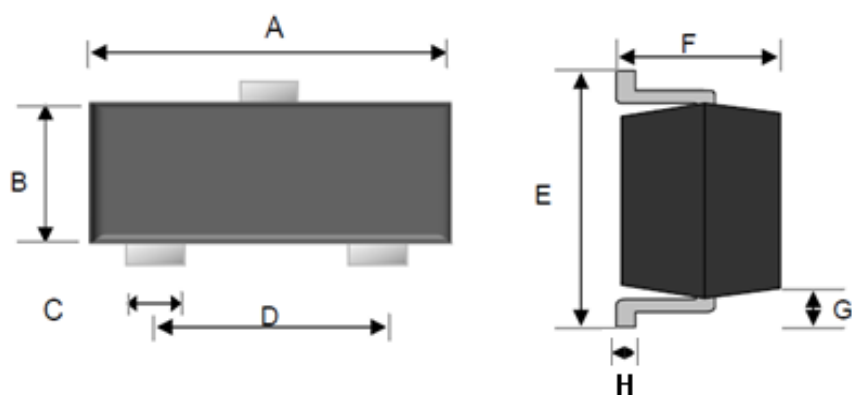
SOT-23
