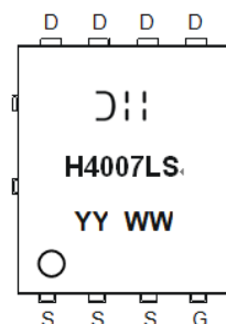
PowerDI5060-8
