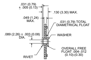
Y Float Mount
