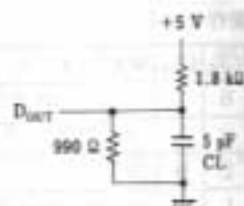
図2. 負荷回路
