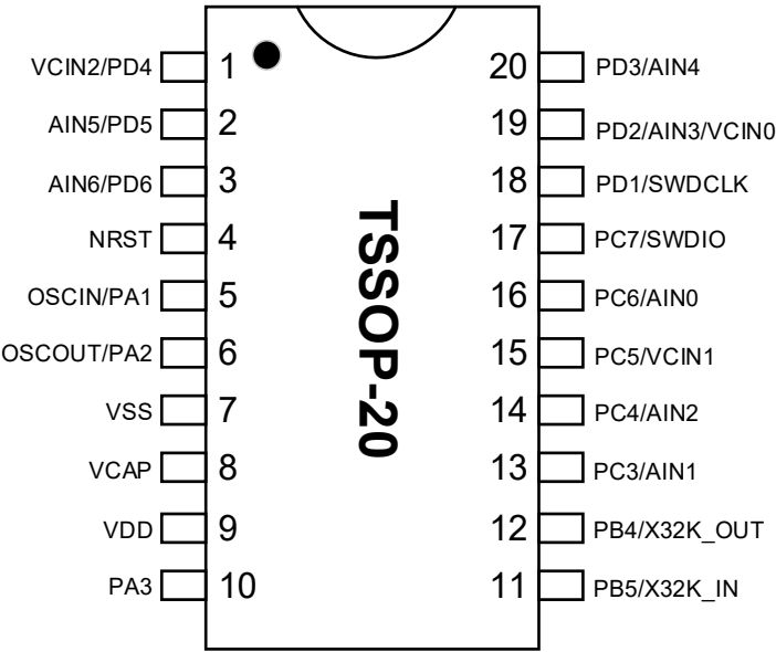
Fig. 4-1 TSSOP20 pin configuration
