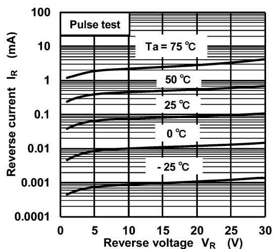
Fig. 8.2 I_R - V_R
