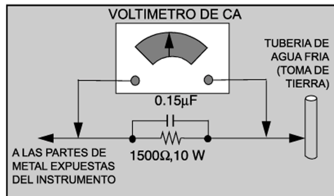
Prueba de circuito con alimentación.
