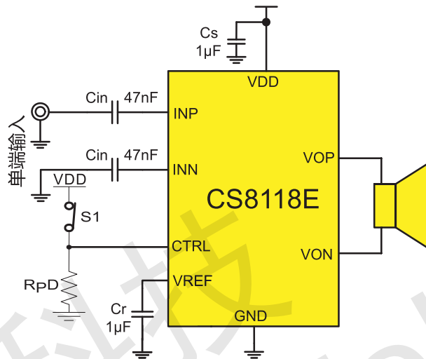
图3 CS8118E单端输入方式应用图(不带防破音)
