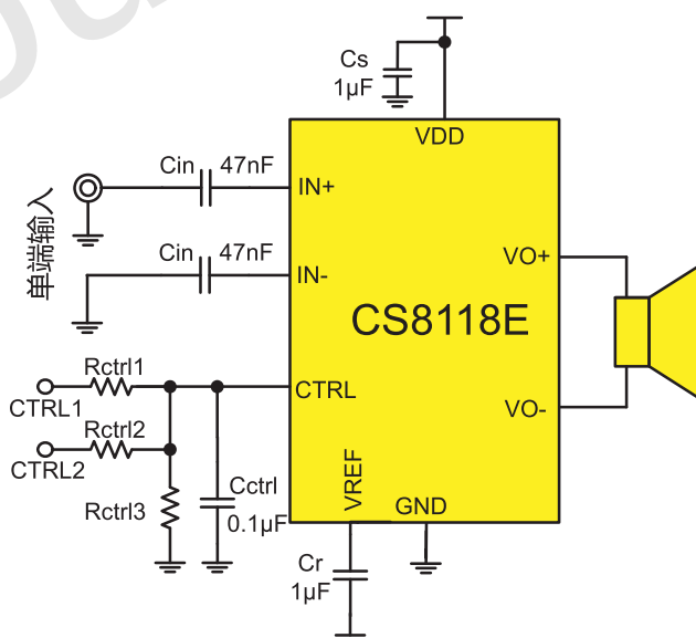
图5 CS8118E单端输入方式应用图(带防破音)
