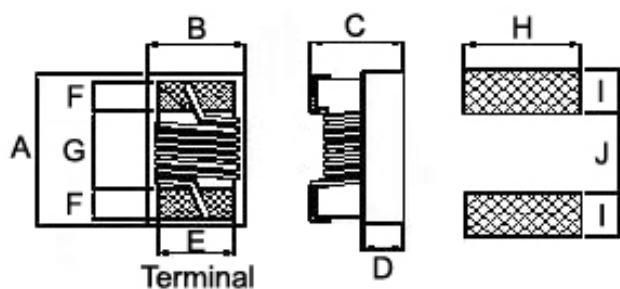
Dimensions
