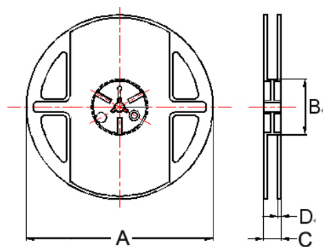
Reel Dimensions
