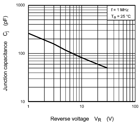
Fig. 10.7 C_j - V_R
