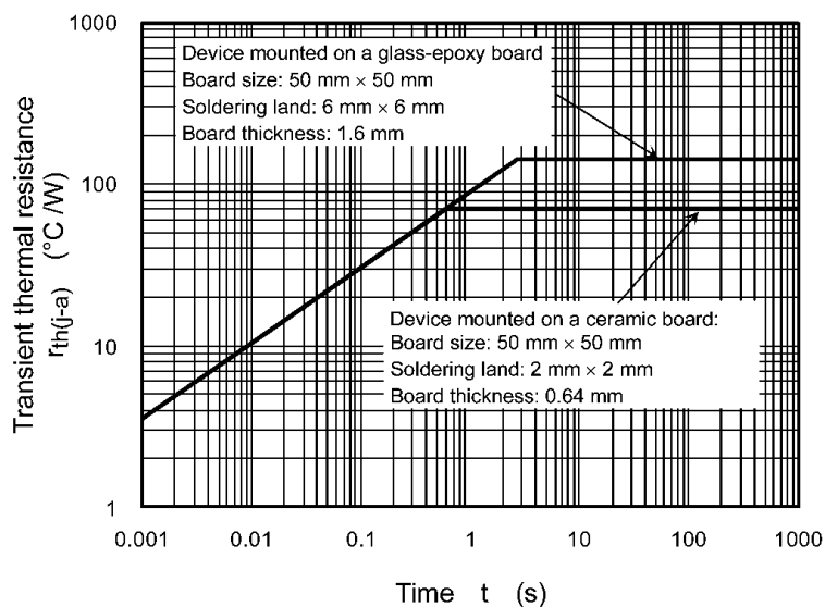
Fig. 10.6 r_{th(j-a)} - t
