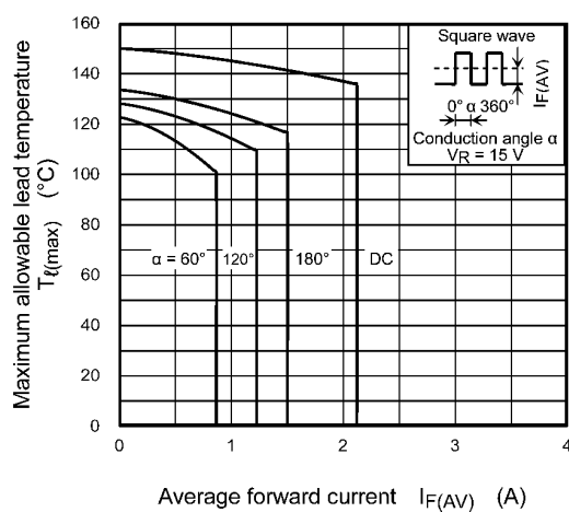
Fig. 10.4 T_{l(max)} - I_{F(AV)}
