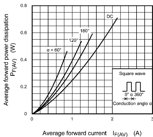
Fig. 10.2 P_{F(AV)} - I_{F(AV)}
