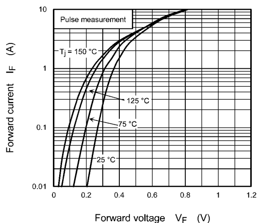
Fig. 10.1 I_F - V_F
