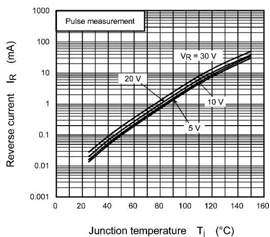
Fig. 10.8 I_R - T_j
