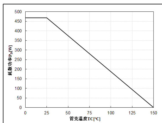
图 17 耗散功率-壳温 T_c 特性 ( T_j \leq 175^\circ\text{C} )
