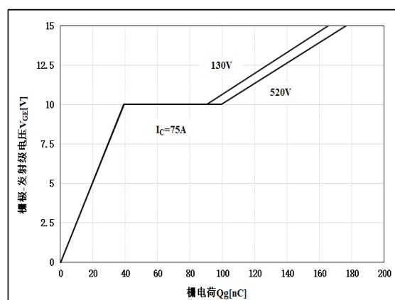
图 18 栅电荷特性
