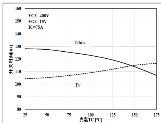
图 10 开通的温度特性
