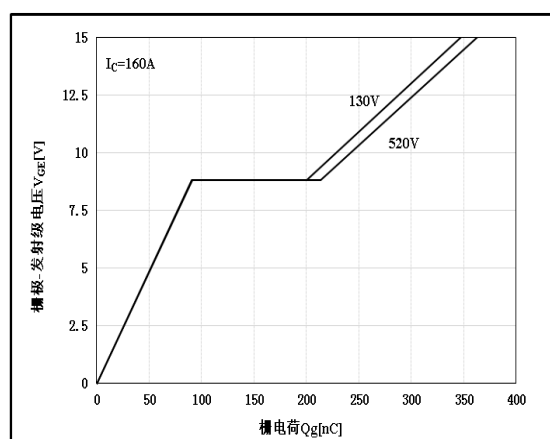
图 18 栅电荷特性
