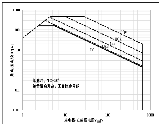
图 19 正向安全工作区
