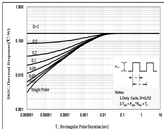
图 20 瞬态热阻特性
