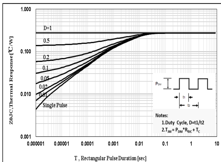
图 20 瞬态热阻特性
