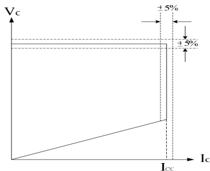
图 1 典型的恒流/恒压曲线
