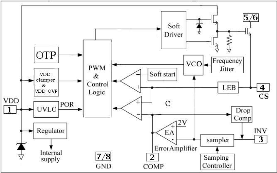
功能框图
