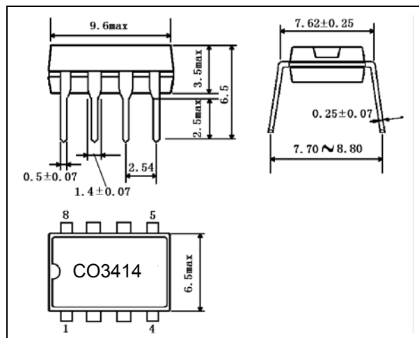
DIP-8
