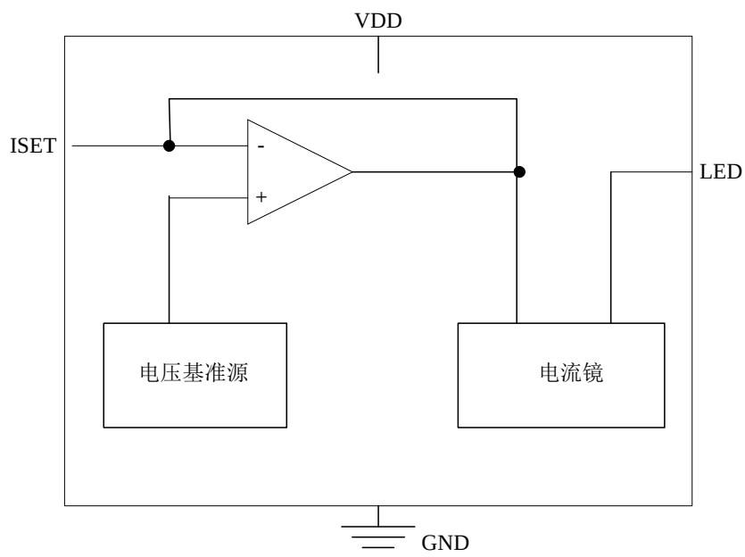
图 2 功能框图
