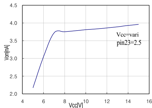
Figure 6. VCC vs. Vom
