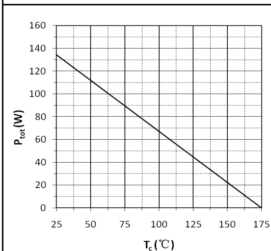
图 5. 功率降额
