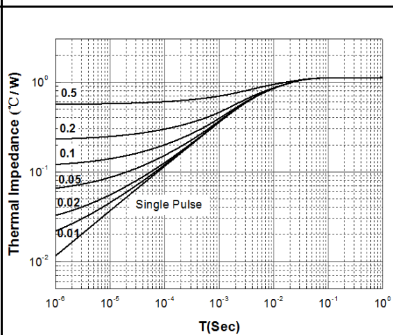
图 6. 瞬态热阻抗
