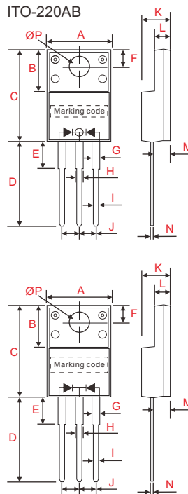
ITO-220AB
