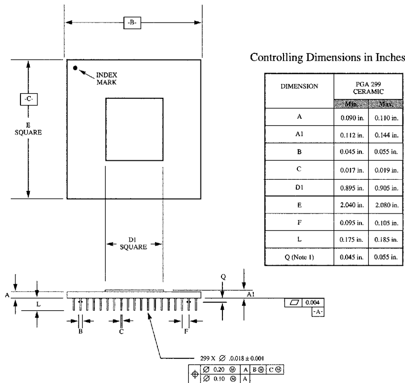
Figure J.1 : 299-pin Cavity-down CPGA Package
