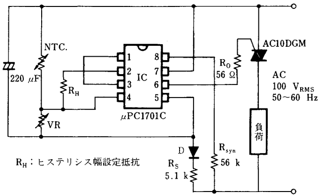
図1 D: オンオフ温度制御回路
