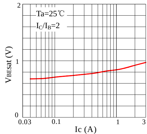
Fig6 VBESat-Ic
