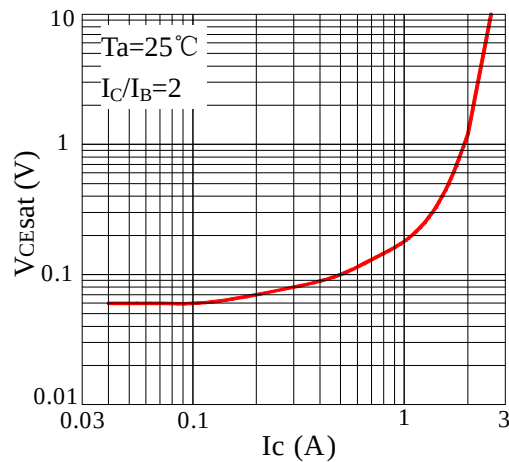
Fig5 VCESat-Ic
