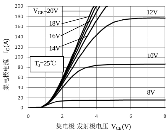
图 1. 输出特性
