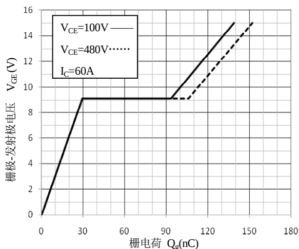
图 14. 栅电荷特性
