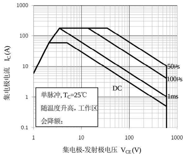
图 12. 安全工作区
