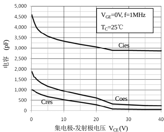
图 7. 电容特性
