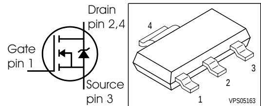
SOT-223
