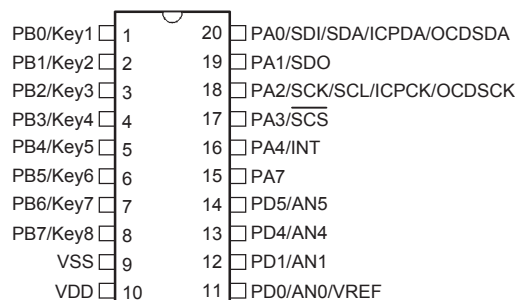
BS84C12A-3/BS84V12A 20 SOP-A/SSOP-A
