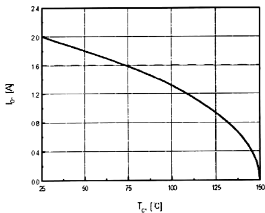
I_D - T_c
