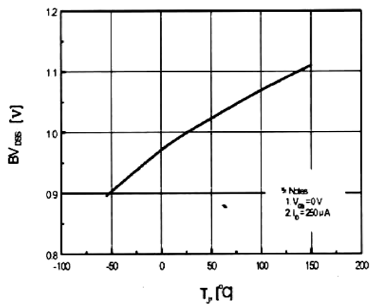
BV_{DSS} - T_J
