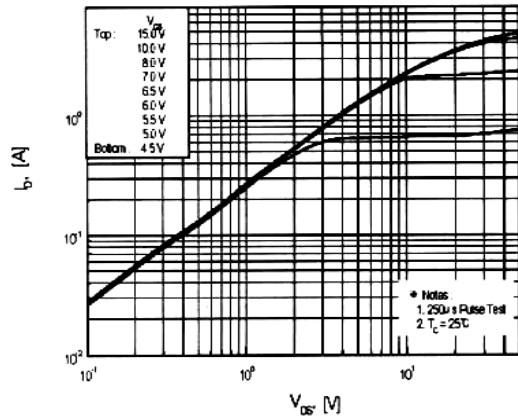
I_D - V_{DS}
