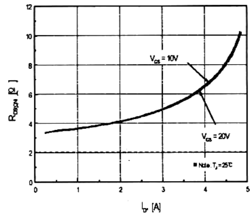
R_{DS(ON)} - I_D
