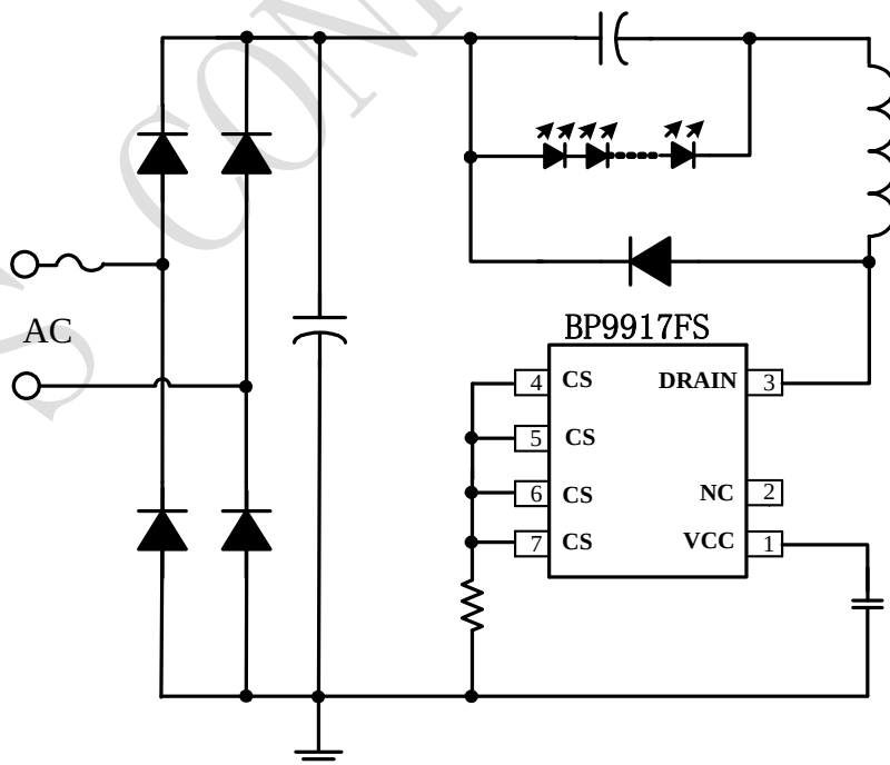
图 1 BP9917FS 典型应用图
