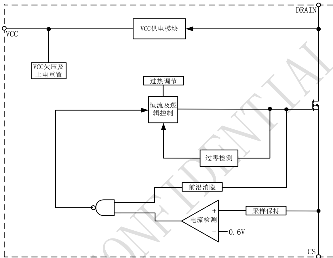
图 3 BP9917FS 内部框图
