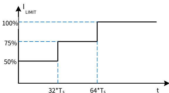
图 6. 软启动过程
