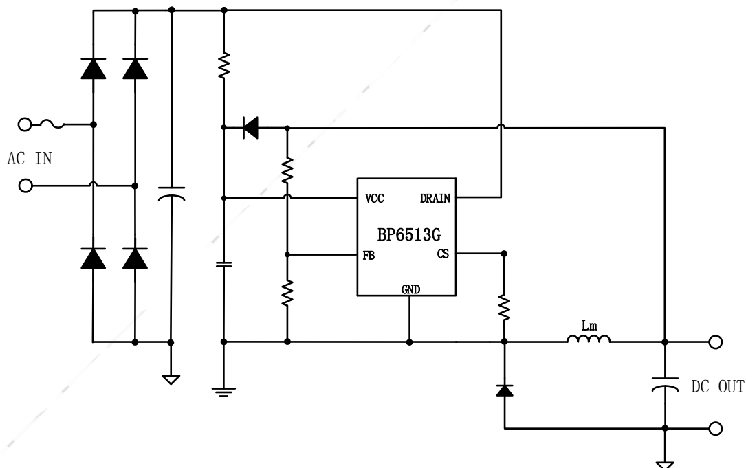
图 1 BP6513G 典型应用图
