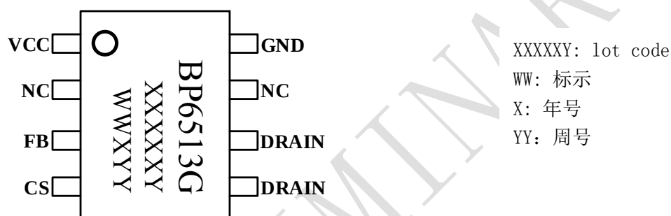
图 2 管脚封装图
