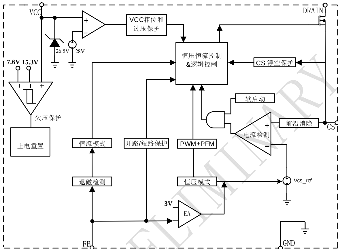
图 3 BP6513G 内部框图
