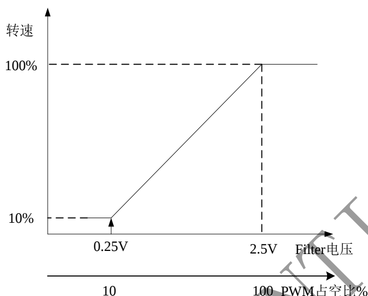
图 6 速度控制范围
