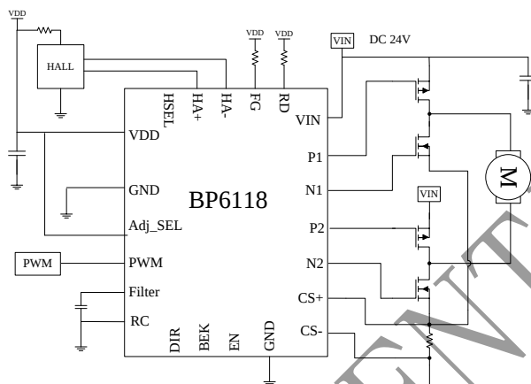
图 5.1 PWM 方波输入调速
