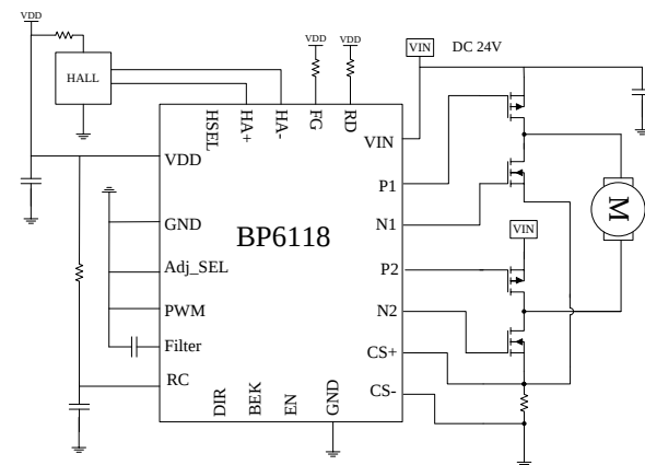
图 5.3 RC 闭环输入调速
