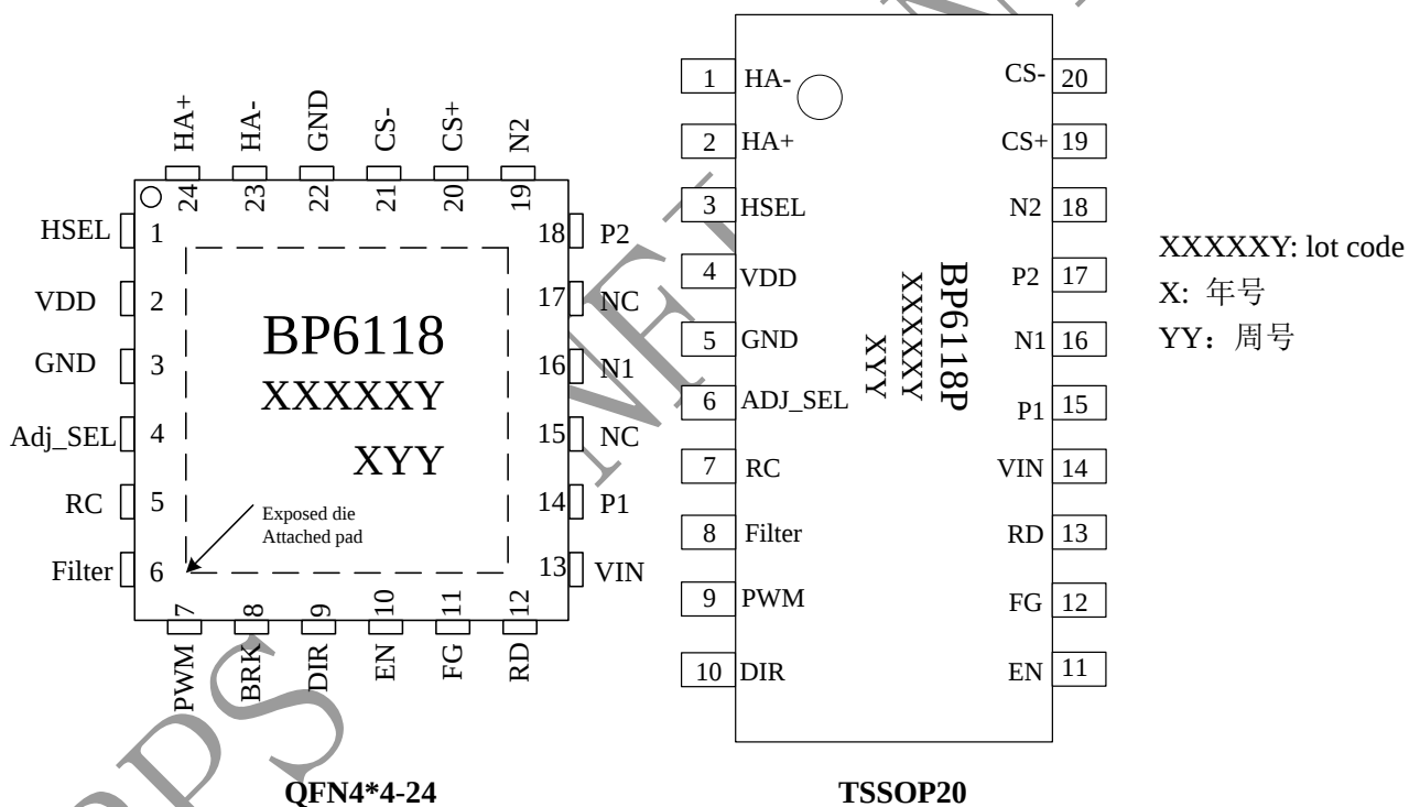
图 2 管脚封装图
