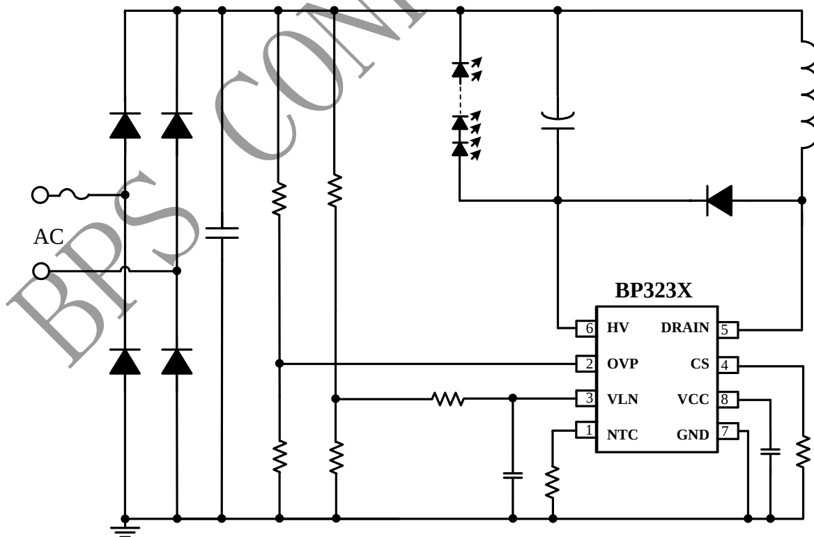
图 1 BP3236H 典型应用图（Buck-Boost）
