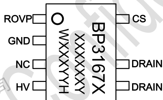
图 2 管脚封装图
