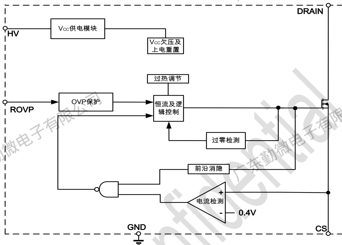
内部结构框图
