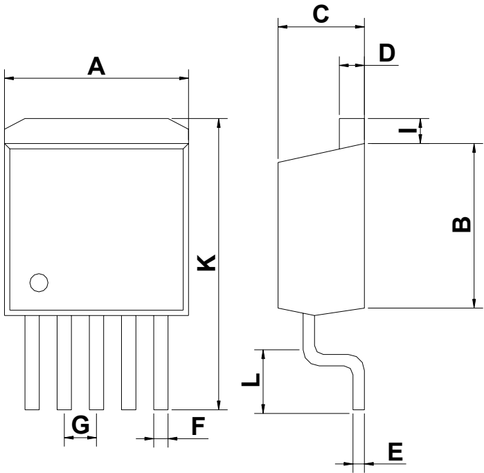
TO-263 (N263)
