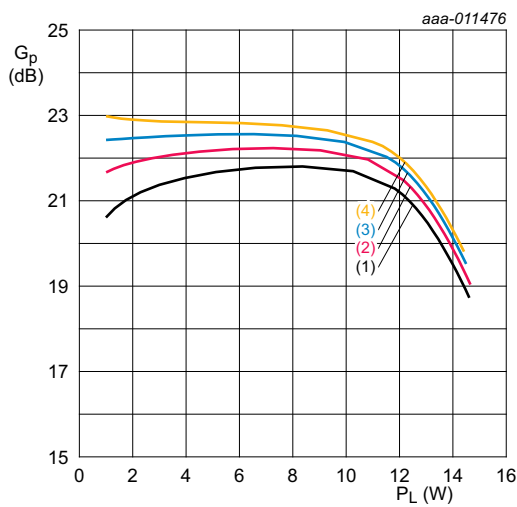
V_{DS} = 50 V; f = 860 MHz. (1) I_{DQ} = 20 mA (2) I_{DQ} = 40 mA (3) I_{DQ} = 60 mA (4) I_{DQ} = 80 mA
