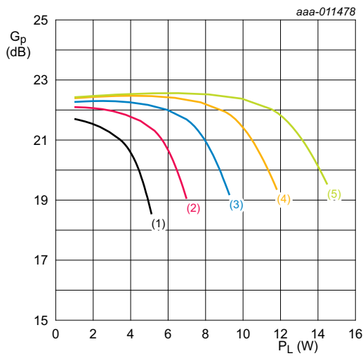
I_{DQ} = 60 mA; f = 860 MHz. (1) V_{DS} = 30 V (2) V_{DS} = 35 V (3) V_{DS} = 40 V (4) V_{DS} = 45 V (5) V_{DS} = 50 V
