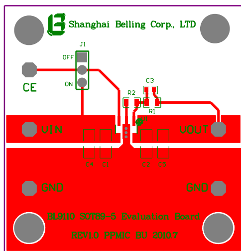
Top Layer
