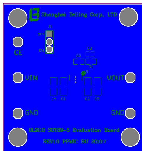
Bottom Layer
