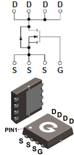
PDFN3×3-8L
