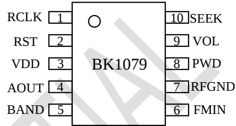
MSOP10 和 SSOP10 管脚定义图（俯视图）
