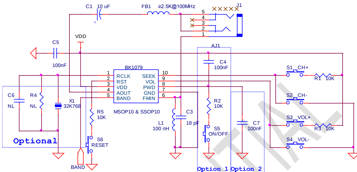
图 2 BK1079 MSOP10 和 SSOP10 应用电路
