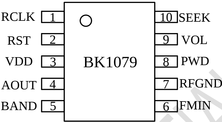
图 1 MSOP10 和 SSOP10 管脚定义俯视图
