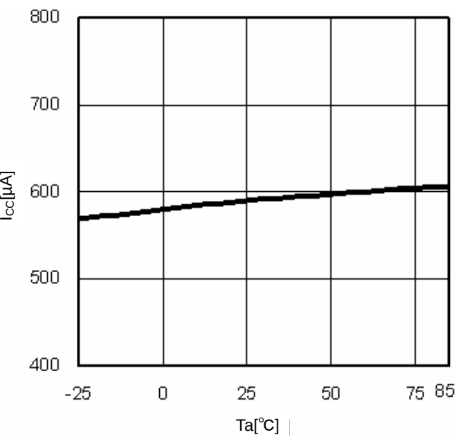
Fig.10 Ta-I CC
