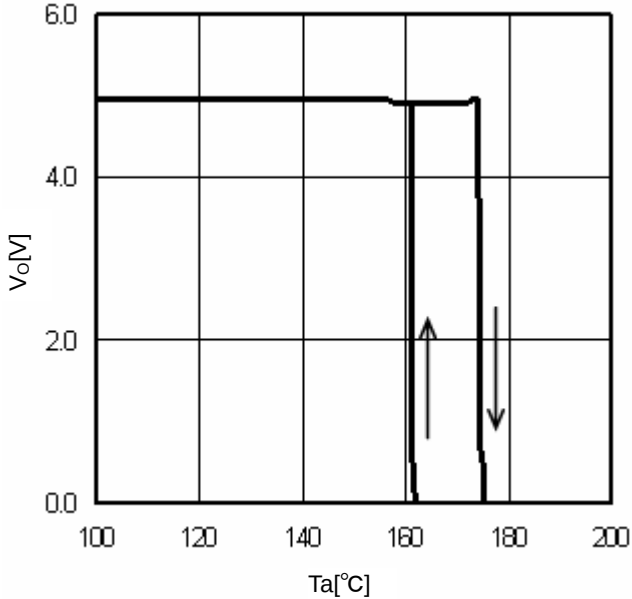
Fig.16 TSD ( I_O=0mA )
