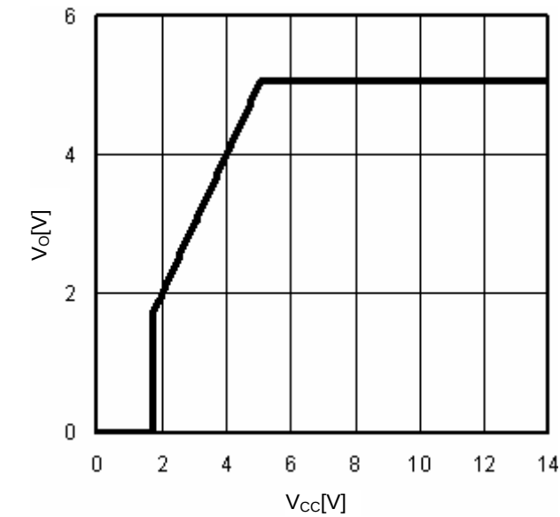
Fig.15 V_{CC}-V_O ( I_O=0mA )
