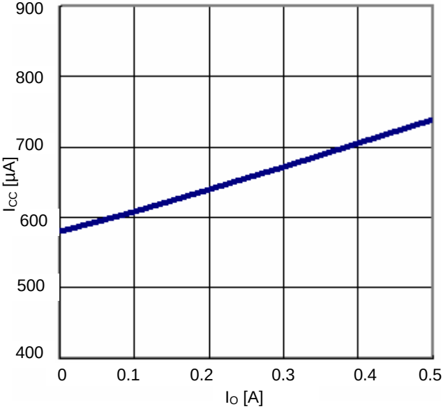
Fig.20 I_o - I_{cc}
