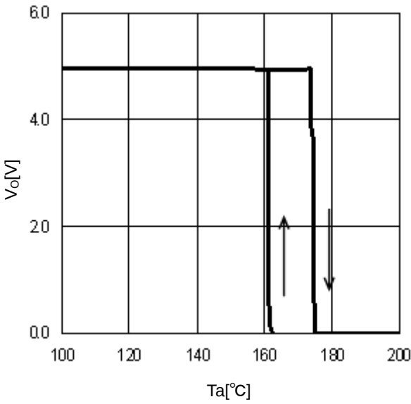
Figure 16. TSD (I O =0mA)
