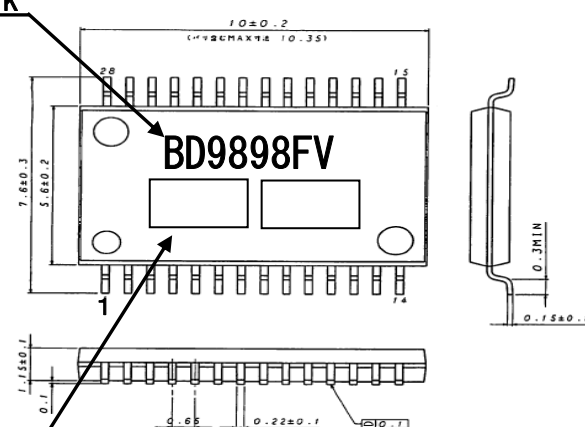
SSOP-B28 (Unit:mm)
