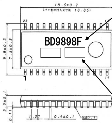
SOP28 (Unit:mm)
