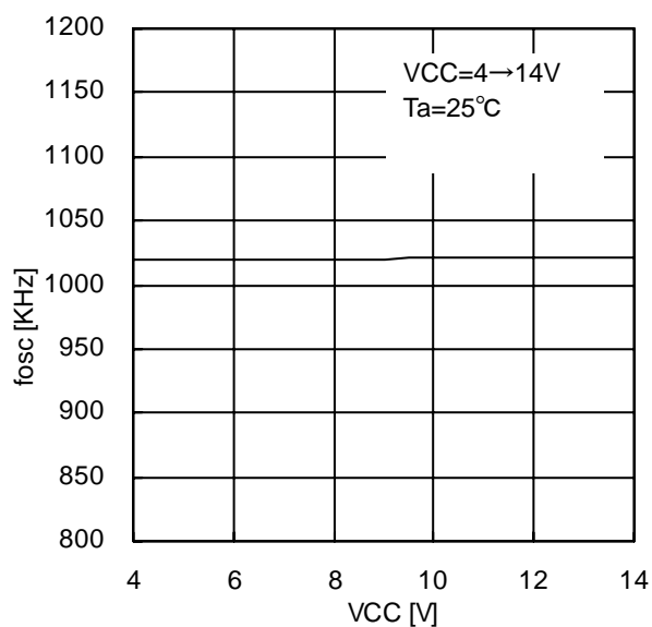
Figure.24 fosc - VCC
